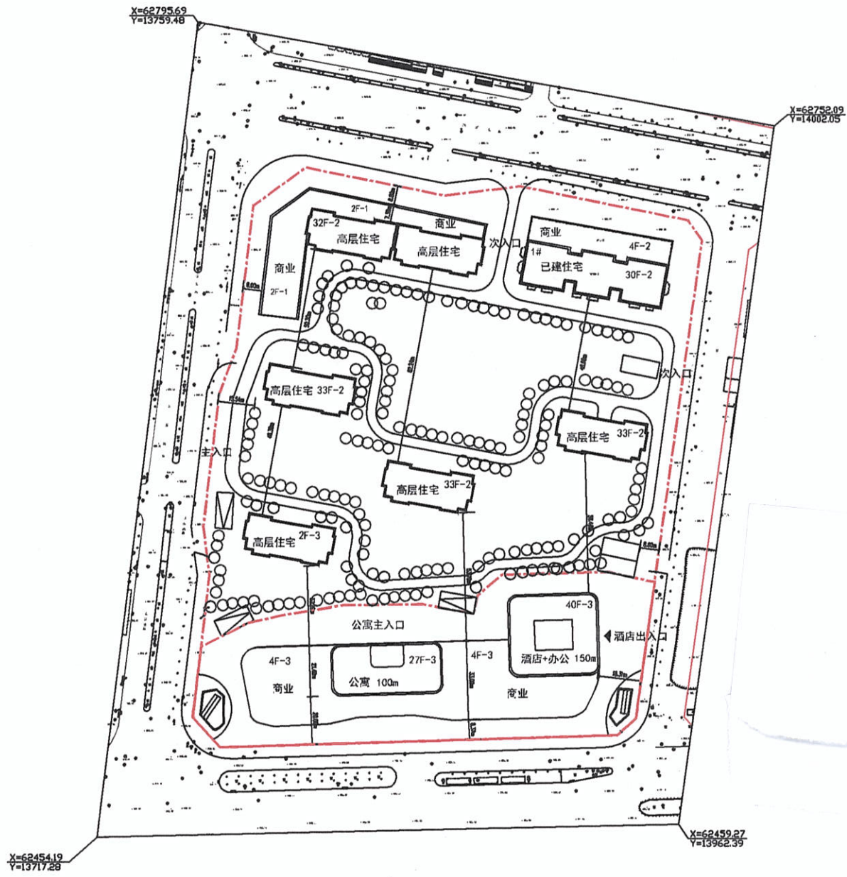
总平面
