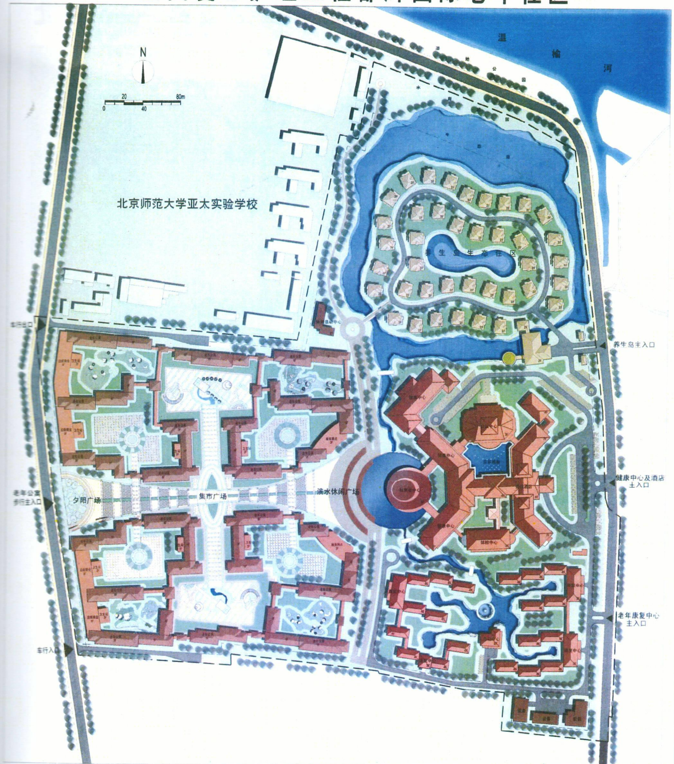
总平面图
