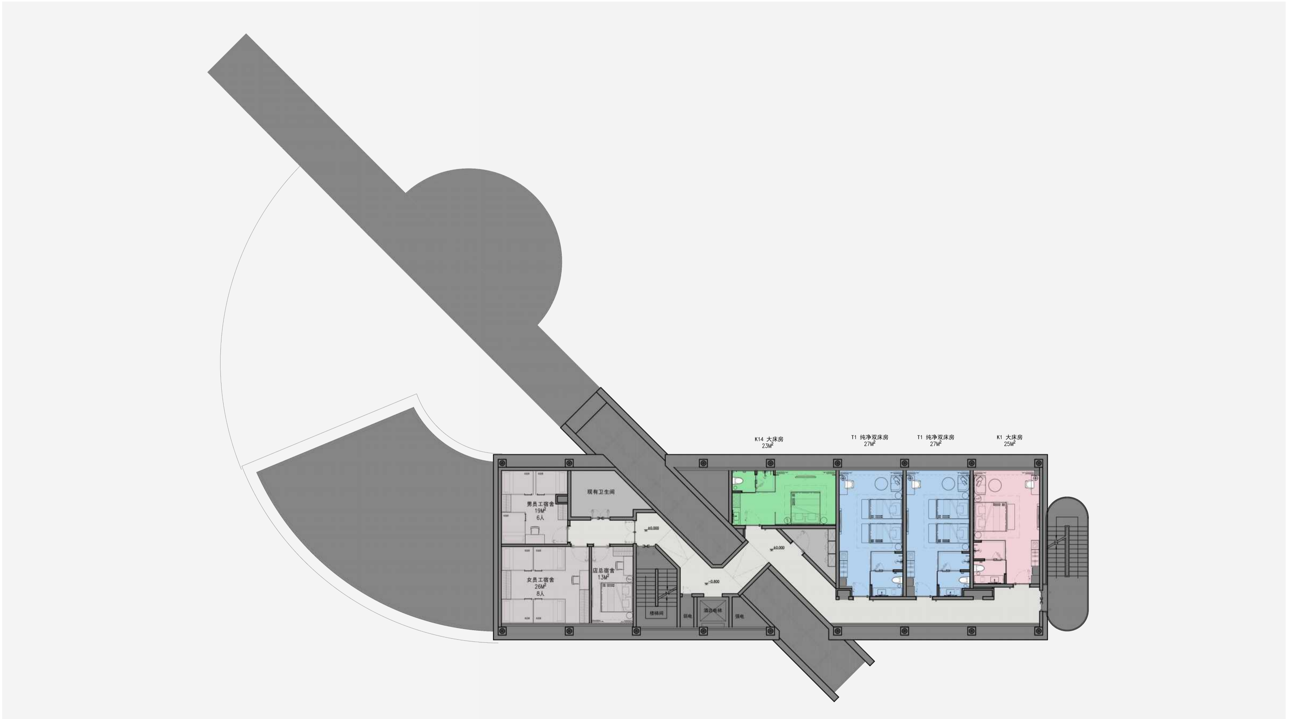
四层夹层平面图
