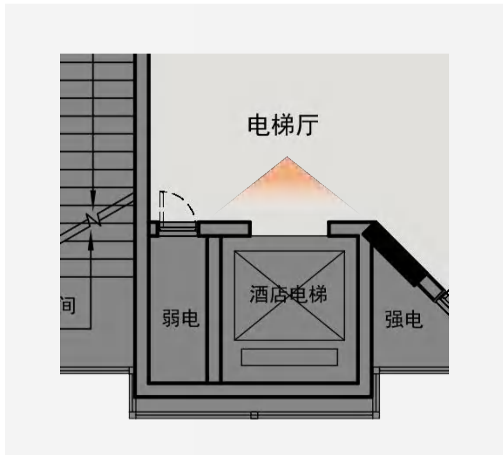
一层平面缩略图
