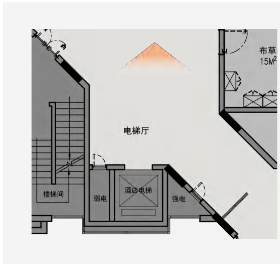
一层至四层夹层平面缩略图
