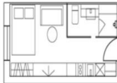
一居室 54平方米户型
